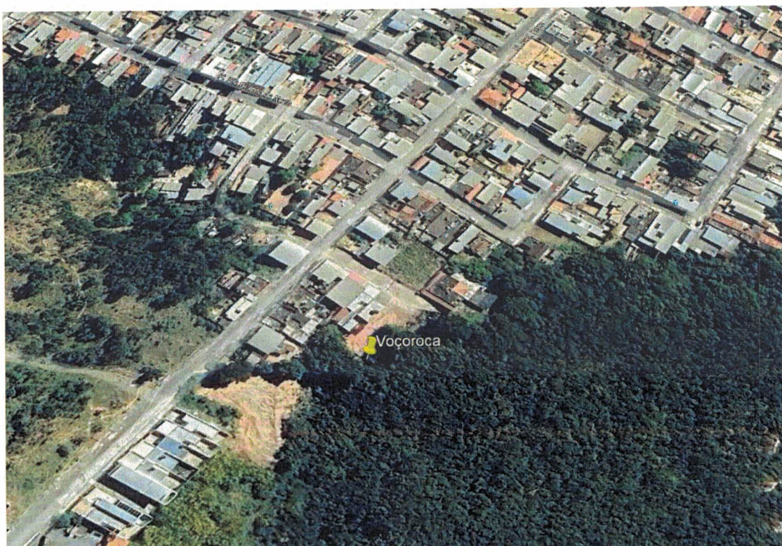
Figura 2 – Localização da voçoroca
