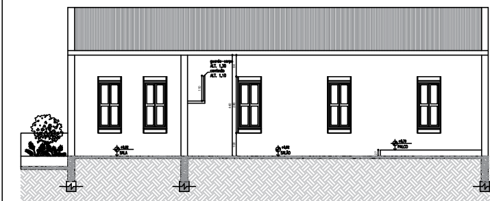
CORTE_B-B escala 1:100
