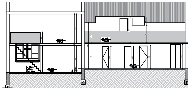
CORTE_A-A escala 1:100
