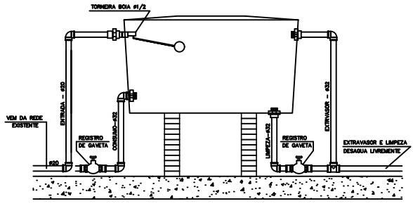
DETALHE ESQUEMATICO - CAIXA D'ÁGUA SEM ESCALA
