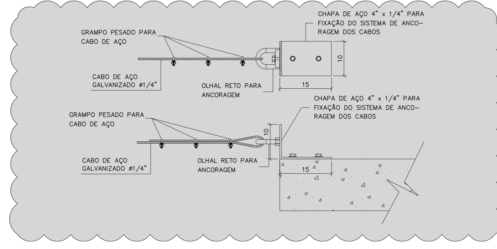
DETALHE 10 - FIXAÇÃO DO CABO DE AÇO ESCALA 1:20
