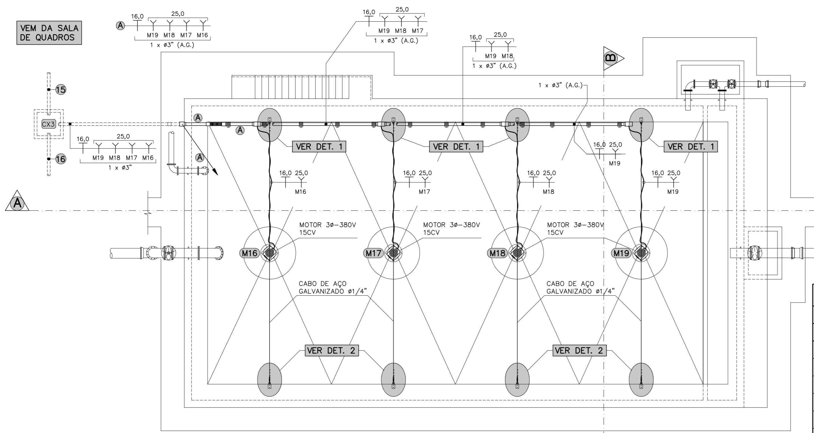
PLANTA BAIXA - AREADOR 4 ESCALA 1:75
