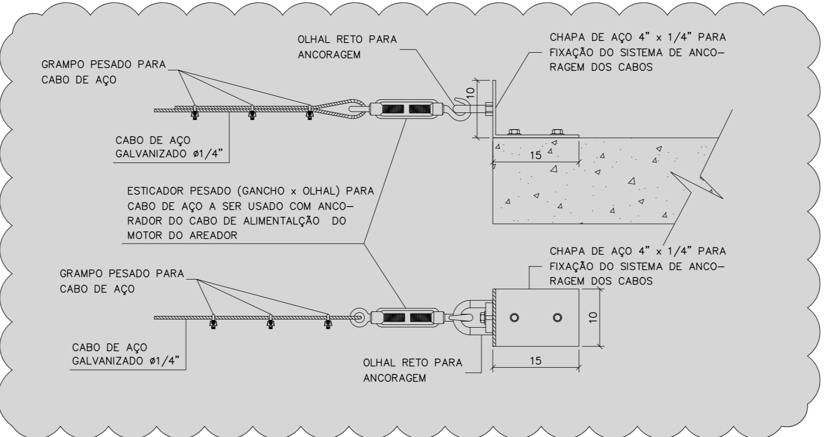
DETALHE 9 - FIXAÇÃO DO CABO DE AÇO ESCALA 1:20
