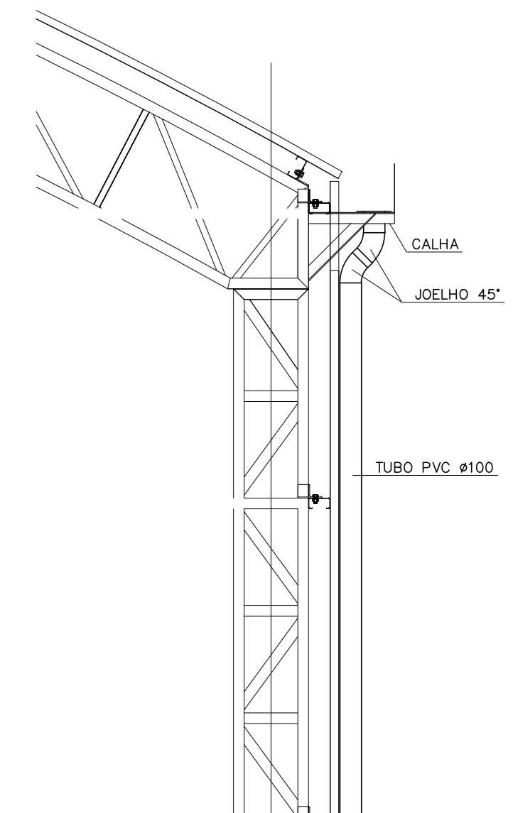
DETALHE DESCIDA DE AGUA SEM ESCALA
