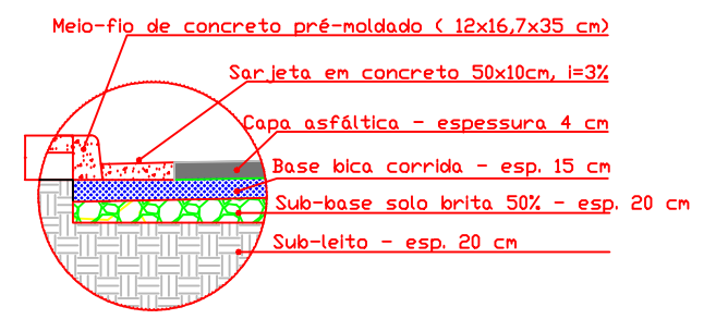
DETALHE 01 - MEIO-FIO E SARJETA SEÇÃO TRANSVERSAL S/ESCALA
