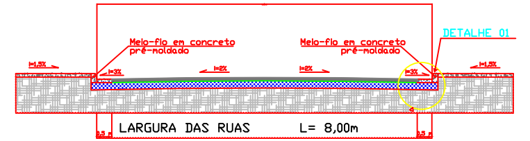
SEÇÃO TÍPICA- IMPLANTAÇÃO ASFÁLTICA S/ESCALA
