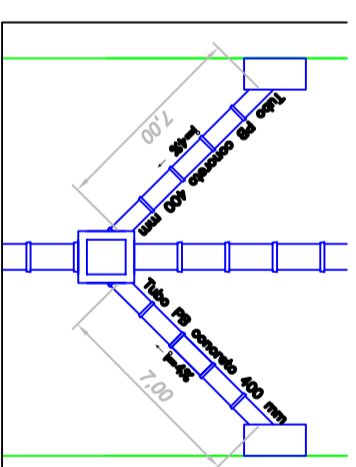
RAMAIS DE LIGAÇÃO SEM ESCALA
